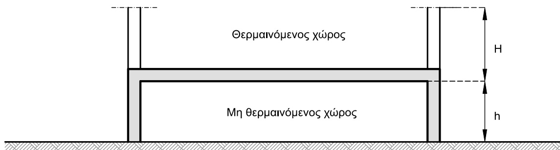
Σχήμα 3. Ενδεικτική διατομή κτηρίου για τον προσδιορισμό του τρόπου υπολογισμού του ισοδύναμου συντελεστή θερμοπερατότητας πλάκας υπερυψωμένης κατά απόσταση h από τη στάθμη του εδάφους.
