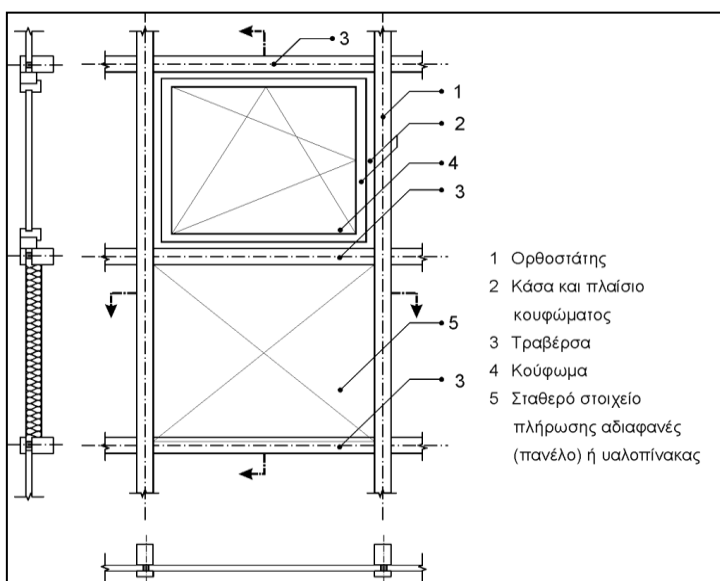
Σχήμα 4. Επιφάνειες τοιχοπετάσματος
