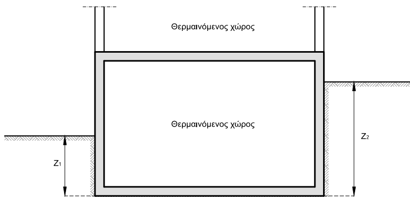
Σχήμα 1. Ενδεικτική διατομή κτηρίου για τον προσδιορισμό του βάθους έδρασης πλάκας επί εδάφους με διαφορετικές στάθμες έδρασης λόγω κεκλιμένου εδάφους.
