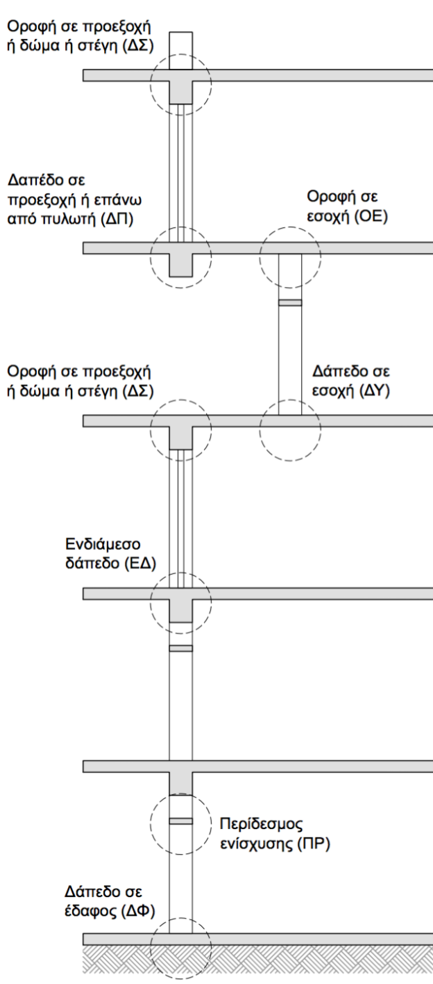
Σχήμα 7. Ενδεικτικές θέσεις εμφάνισης οριζόντιων θερμογεφυρών.
