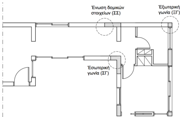
Σχήμα 6. Ενδεικτικές θέσεις εμφάνισης κατακόρυφων θερμογεφυρών.
